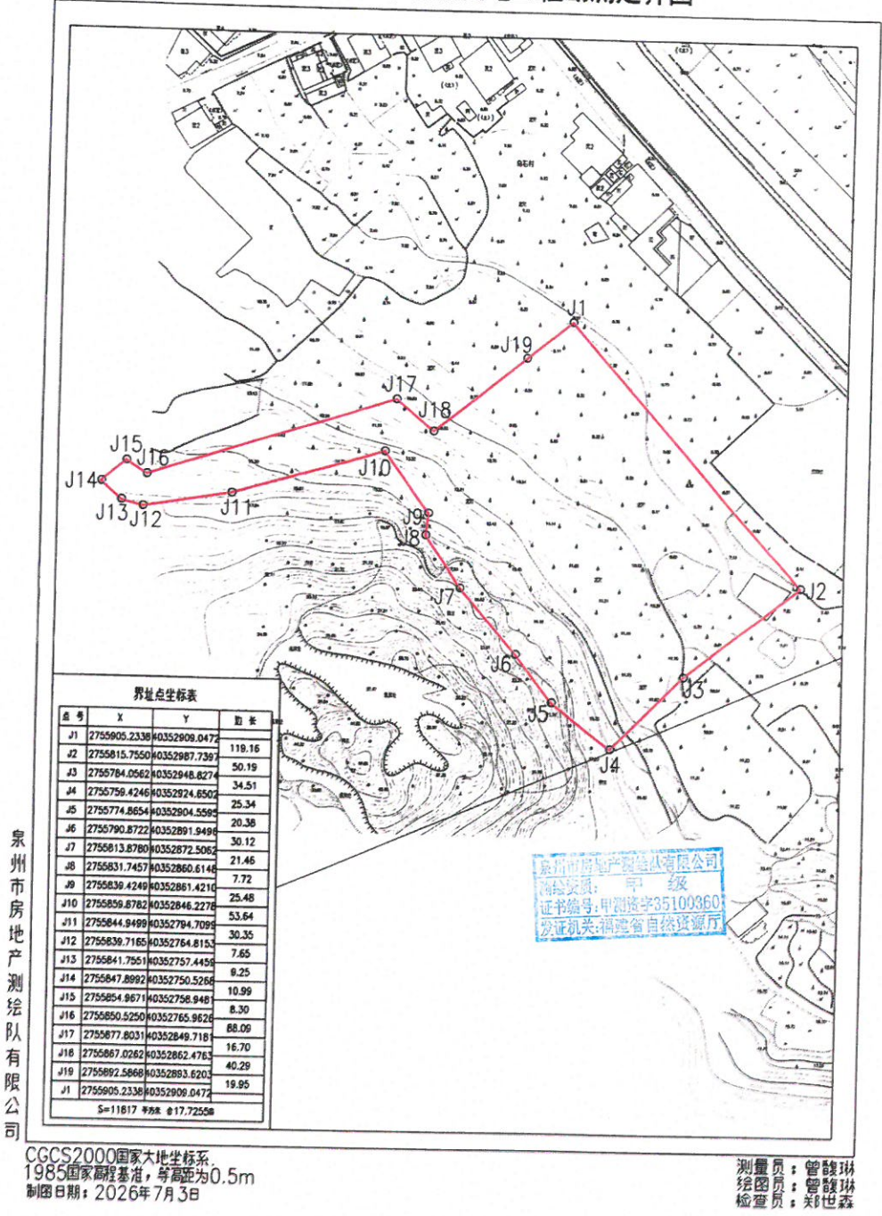
泉州玉霞220千伏输变电工程勘测定界图
